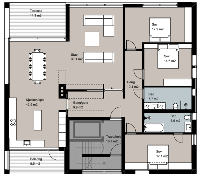
HUS C - Leilighet 3.1 - 167,7 m 2 BRA-i
