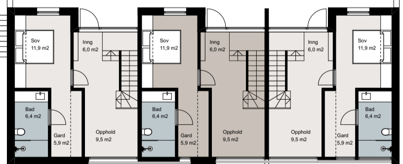
HUS E - Rekkehus 1
