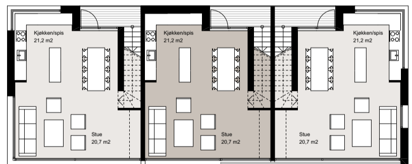
HUS E - Rekkehus 1
